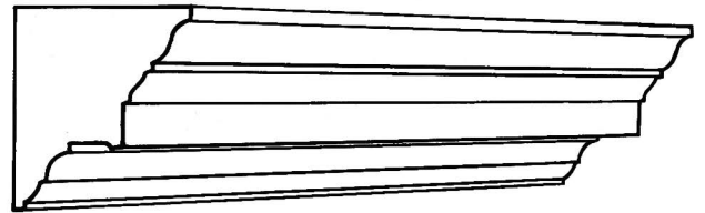
CP143 Projection 108mm(4 1 / 4 ") Depth 125mm(5")
