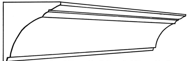
CP107 Projection 112mm(4 3 / 8 "") Depth 117mm(4 5 / 8 "")
