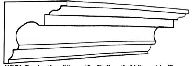
CP71 Projection 90mm(3 1 / 2 ") Depth 108mm(4 1 / 4 ")
