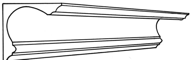
CP 109 Projection 115mm(4 1 / 2 "") Depth 115mm(4 1 / 2 "")
