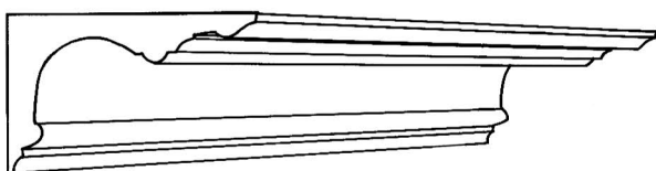
CP198 Projection 190mm(7 1/2") Depth 120mm(4 3/4")
