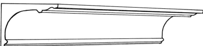
CP208 projection 125mm( 4\frac{7}{8} "") depth 98mm( 3\frac{7}{8} "")
