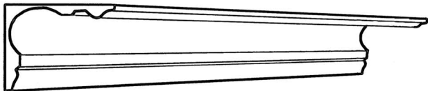
CP124 Projection 140mm(5 1 / 2 "") Depth 110mm(4 3 / 8 "")
