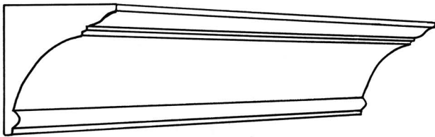
CP132 Projection 120mm(43/4") Depth 143mm(51/2")
