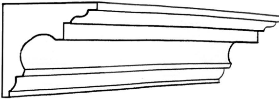
CP72 Projection 114mm(4 1 / 2 ") Depth 114mm(4 1 / 2 ") CP72a Projection 128mm(5") Depth 128mm(5")
