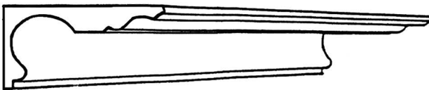
CP76 Projection 121mm(4 3 / 4 ") Depth 67mm(2 5 / 8 ")
