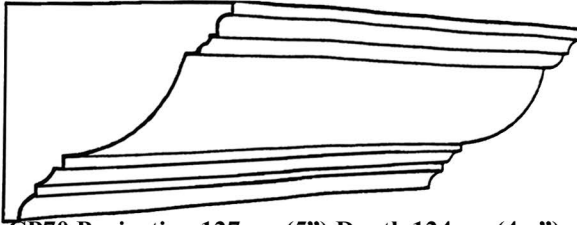
CP70 Projection 127mm(5") Depth 124mm(4 7 / 8 ")
