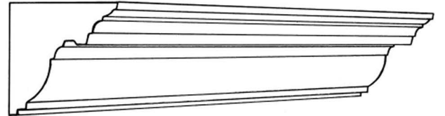
CP205 projection 118mm( 4\frac{5}{8} "") depth 125mm( 4\frac{7}{8} "")
