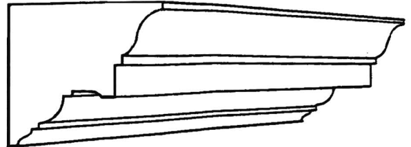
CP53 Projection 102mm(4") Depth 89mm(3 1/2")
