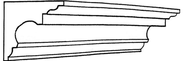
CP73 Projection 153mm(6") Depth 153mm(6")
