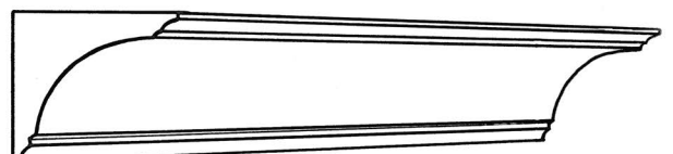
CP159 Projection 114mm(4 1 / 2 "") Depth 100mm(4"")
