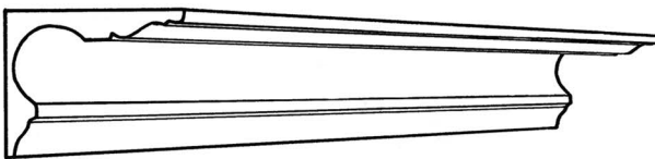
CP166 Projection 145mm(5 5 / 8 "") Depth 115mm(4 5 / 8 "")
