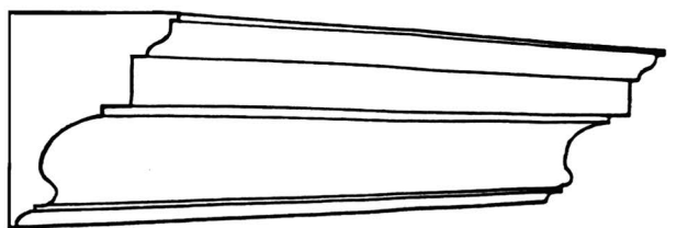
CP69 Projection 95mm(3 3/4") Depth 111mm(4 3/8")
